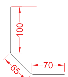
D260 WALL FILLET TRIM 902702
