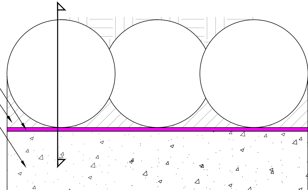
SECANT PILE PLAN
